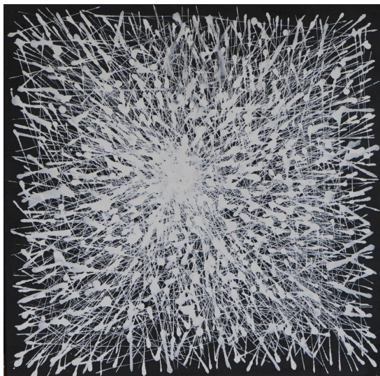
Kollisionen einiger Myonen
